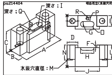
138_切出水鉢
