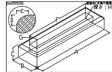
250_墓誌/01_墓誌台
