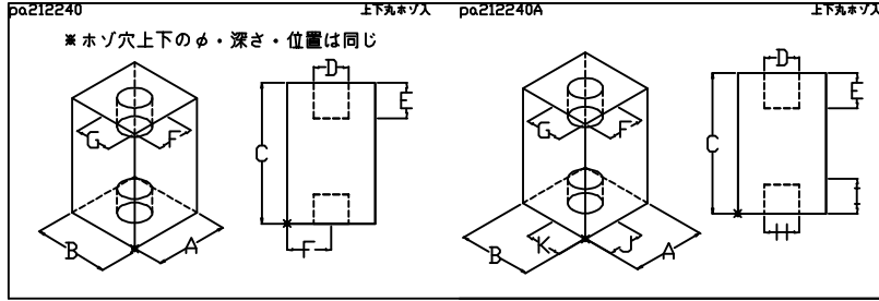
001_親柱 / 03_前面傾斜型
